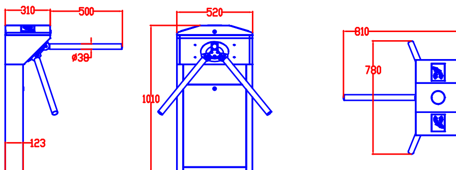
TORNELLO TRIPODE
